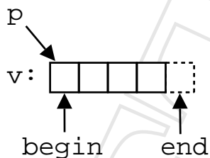
Фиг. 1. Указатели и масиви
