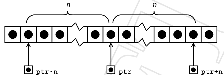
Фиг. 2. Аритметика с указатели: събиране и изваждане на цяло число и указател
