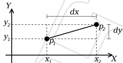
Фиг. 5. Разстояние между две точки в равнината
