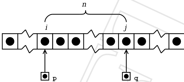
Фиг. 4. Аритметика с указатели: изваждане на указатели
