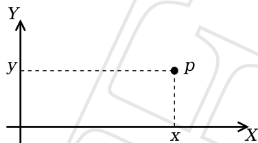
Фиг. 6. Декартови координати на точка в равнината
