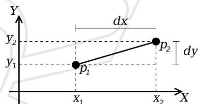
Фиг. 7. Разстояние между две точки в равнината
