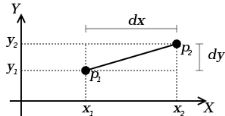
Фиг. 5. Разстояние между две точки в равнината
