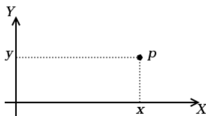
Фиг. 6. Декартови координати на точка в равнината
